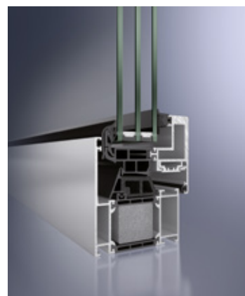
Schüco AWS 75 BS.SI+ Anta coperta con sezione in vista ridotta (sistema tipo "Block") Schüco AWS 75 BS.SI+ Concealed vent with narrow face width (block system)
