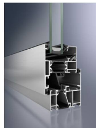
Schüco AWS 65 TipTronic, apribile verso l'esterno, con guarnizione centrale (anta rotante a sporgere, finestra a sporgere) Schüco AWS 65 TipTronic, outward-opening, with centre gasket (projected side-hung, projected top-hung)
