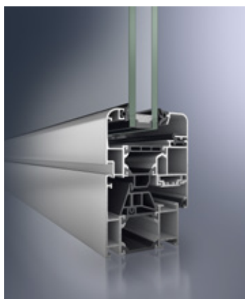
Schüco AWS 65 SL Contorno esterno arrotondato (Soft Line Contour) Schüco AWS 65 SL Rounded external contour (Soft Line contour)
